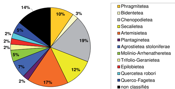
Fig. 24 : Toul (54) « Secteur Vauban intra muros », suivi de travaux, Inrap 2012. Secteur 17 « Place de la Croix de Fûe ». Répartition des classes syntaxinomiques représentées par les taxons* de plantes sauvages (DAO : J. Wiethold, Inrap).
