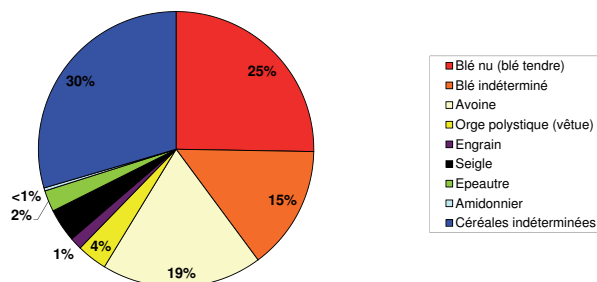
Fig. 20 : Toul (54) « Secteur Vauban intra muros », suivi de travaux, Inrap 2012. Secteur 23 « Place Dr. Pierre Schmidt ». Répartition des caryopses et de céréales (n = 281) dans les prélèvements de l'u.s. 231042 (DAO : J. Wiethold, Inrap).
