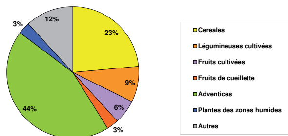
Fig. 19 : Toul (54) « Secteur Vauban intra muros », suivi de travaux, Inrap 2012. Secteur 23 « Place Dr. Pierre Schmidt ». Répartition des taxons par classe fonctionnelle (n=34) dans les prélèvements de l'u.s. 231042 (DAO : J. Wiethold, Inrap).
