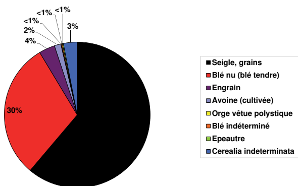
Fig. 28 : Toul (54) « Secteur Vauban intra muros », suivi de travaux, Inrap 2012. Secteur 31 « Rue du Pont de Vaux ». Répartition des caryopses et de céréales (n = 7749) dans le prélèvement de l'u.s. 311020 (DAO : J. Wiethold, Inrap).
