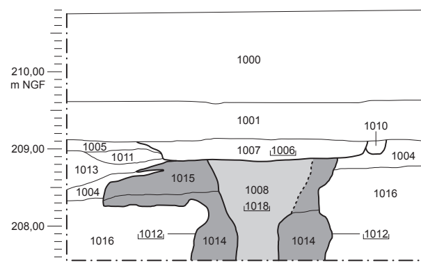
Fig. 5 : Toul (54) « Secteur Vauban intra muros », suivi de travaux, Inrap 2012. Secteur 08, rue Chanzy. Le fossé s'est formé sur plus de 1,20 m de profondeur (DAO : R. Jude, Inrap).
