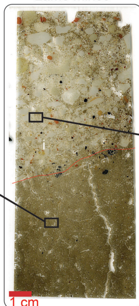
Fig. 17 : Analyse micromorphologique, faciès des US 103 et 104 (© Carole Vissac – Géoarchéon).
