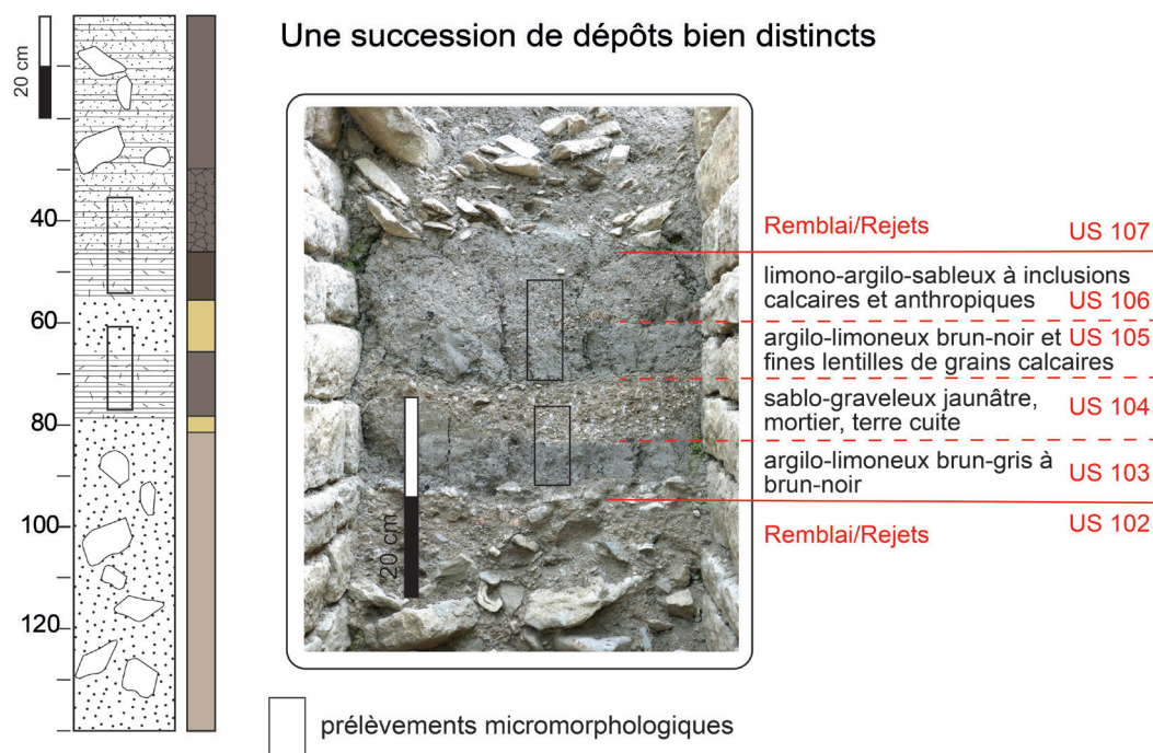
Fig. 7 : Grand - Rue du Ruisseau (Vosges). Caractères macroscopiques des US de la canalisation et localisation des prélèvements micromorphologiques (© Carole Vissac – Géoarchéon).
