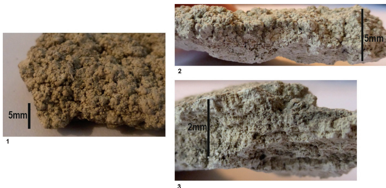
Fig. 13 : Photographies des faciès d'encroûtements carbonates du type „choux-fleurs“. 1 Vue sommitale (face inférieure d'une assise). 2 Vue latérale (structure en colonnes de rhomboèdres). 3 Vue latérale (succession de lamines à colonnes). Les échelles sont approximatives (@ Julie Dabkowski -Géoarchéon).
