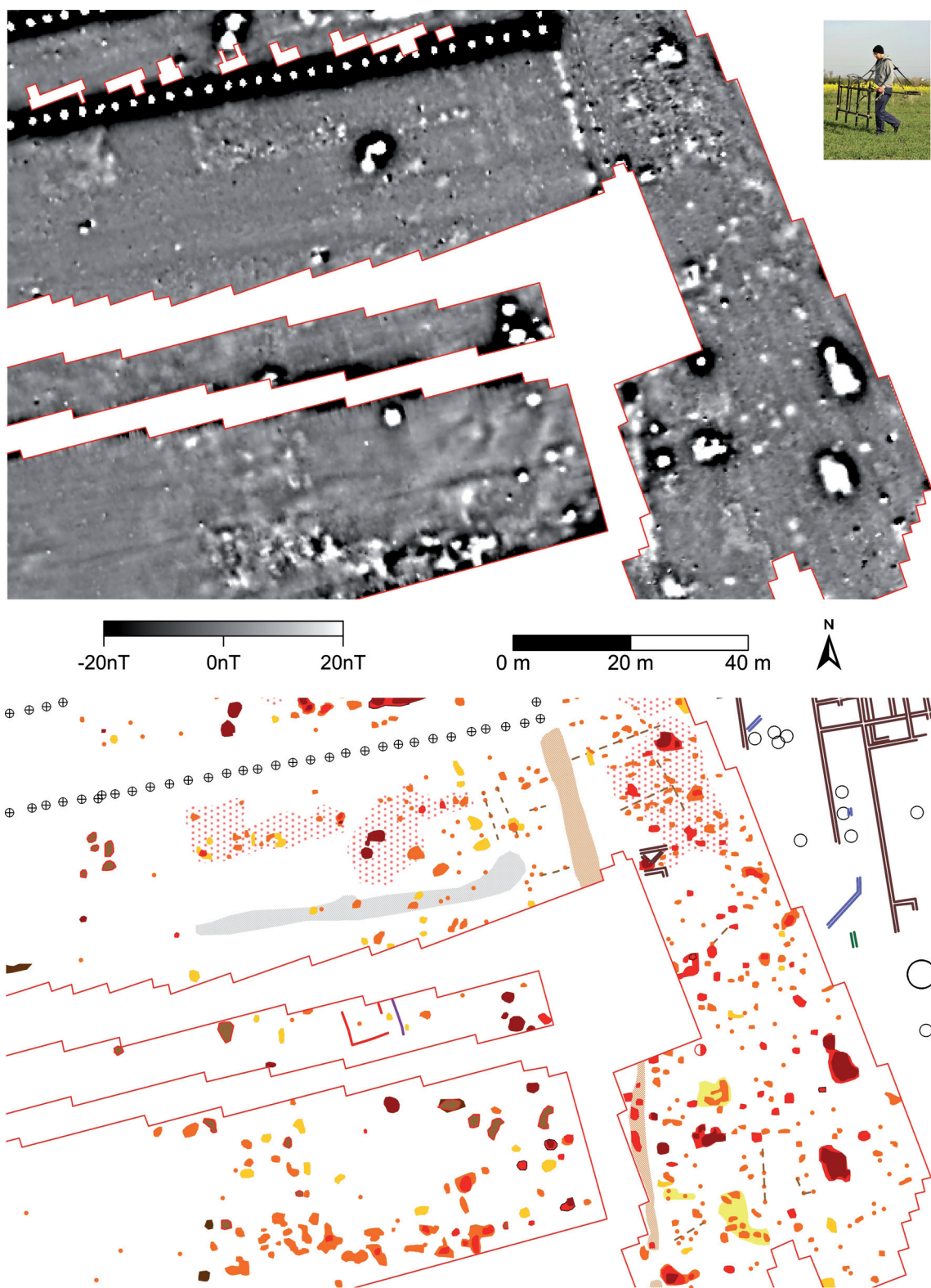
Abb. 5: Römischer vicus, Mamer, Luxembourg, Detail der Graustufendarstellung der Magnetometerprospektion und Interpretation [Grafik: PZP GbR im Auftrag des Centre national de recherche archéologique, Bertrange, Luxembourg; Foto: PZP GbR].
