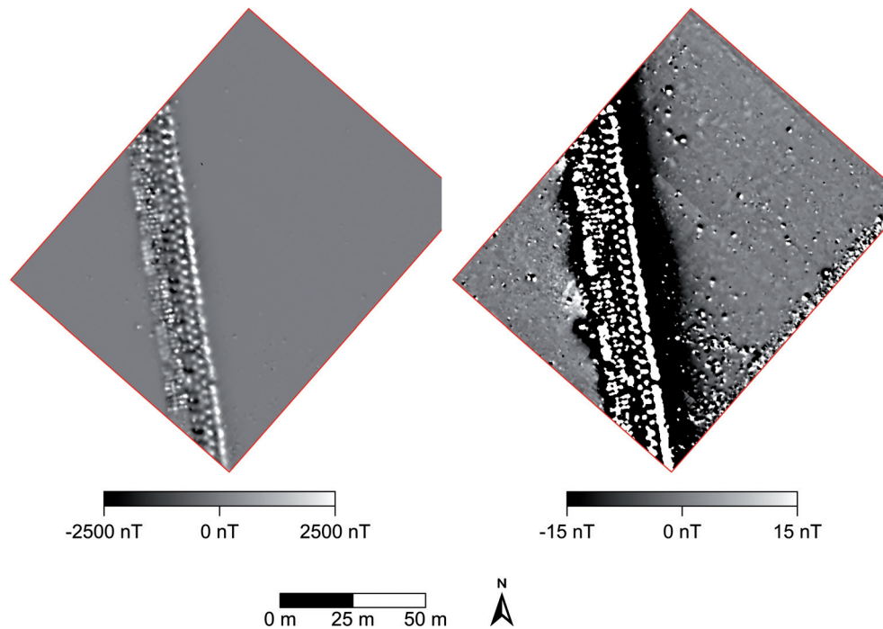
Abb. 8: Panzersperre des „Westwalles“, Vinningen, Verbandsgemeinde Pirmasens-Land, Landkreis Südwestpfalz, Detail der Graustufendarstellung der Magnetometerprospektion mit unterschiedlichen Messwertbereichen [Grafik: PZP GbR im Auftrag der juwi Energieprojekte GmbH, Wörrstadt].
