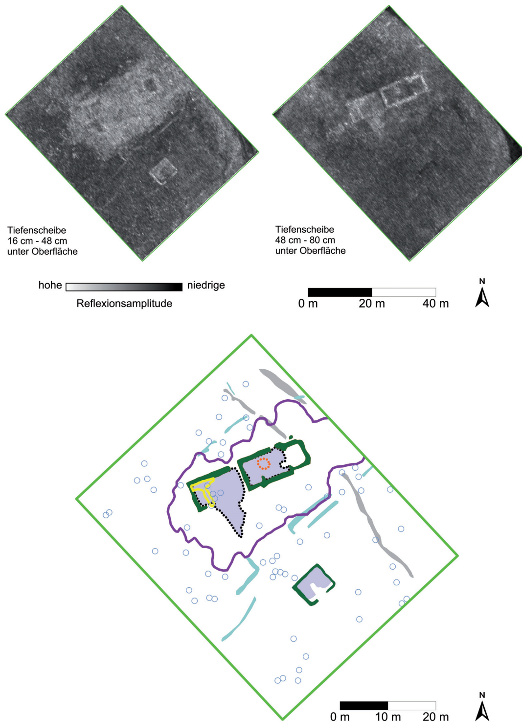
Abb. 7: Kirchengrundriss, Klosterwüstung, Bad Berleburg-Wunderthausen, Kreis Siegen-Wittgenstein, Graustufendarstellung zweier Tiefenscheiben der Bodenradarprospektion und Interpretation [Grafik: PZP GbR im Auftrag des Kriegervereines Wunderthausen - Traditionsverein, Bad Berleburg].
