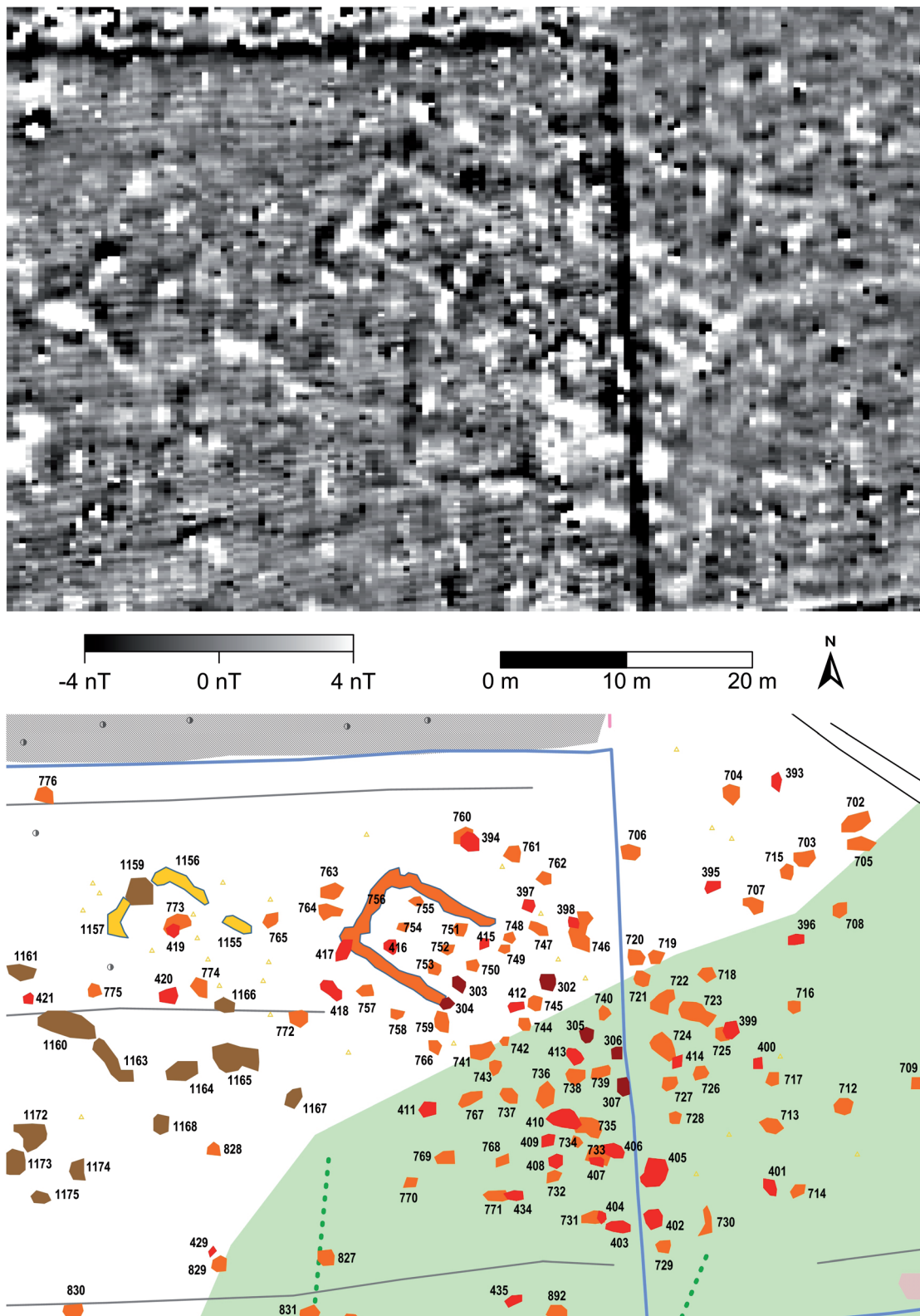
Abb. 1: Neolithische Siedlung, Frisange und Weiler-la-Tour, Luxembourg, Detail der Graustufendarstellung der Magnetometerprospektion und Interpretation [Grafik: PZP GbR im Auftrag des Centre national de recherche archéologique, Bertrange, Luxembourg].
