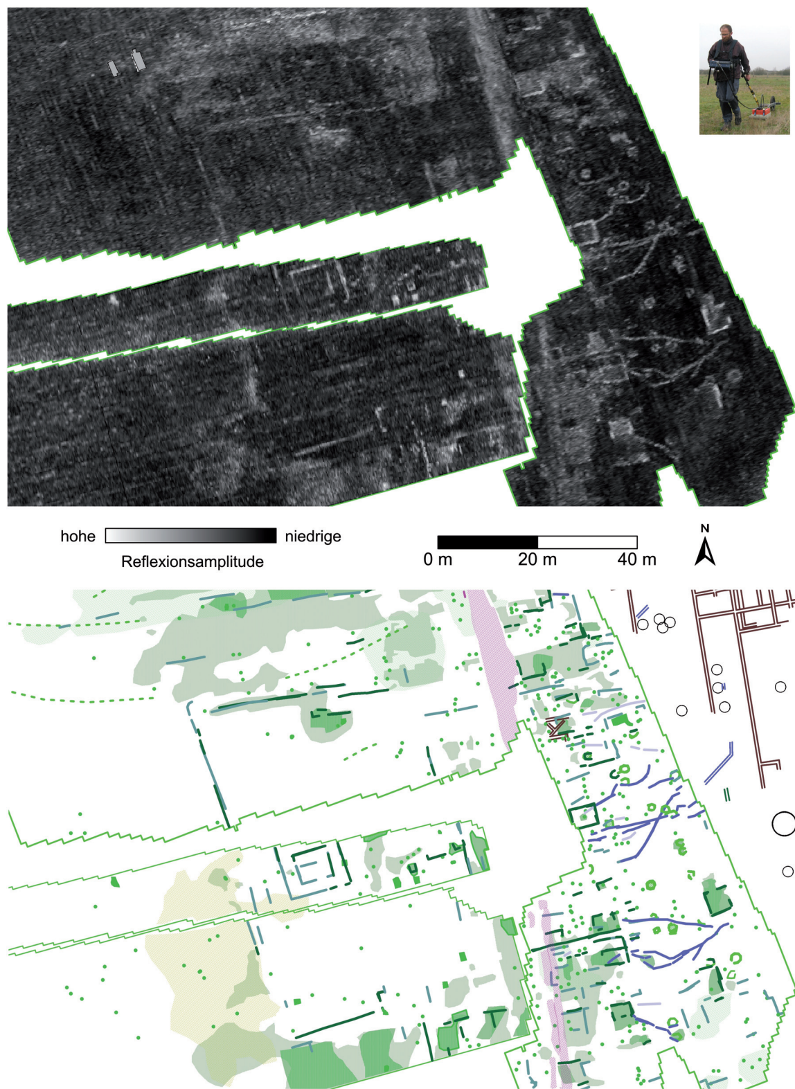
Abb. 6: Römischer vicus, Mamer, Luxembourg, Detail der Graustufendarstellung einer Tiefscheibe des Bodenradars (0,25 m bis 0,5 m unter Oberfläche) und Interpretation [Grafik: PZP GbR im Auftrag des Centre national de recherche archéologique, Bertrange, Luxembourg; Foto: PZP GbR].
