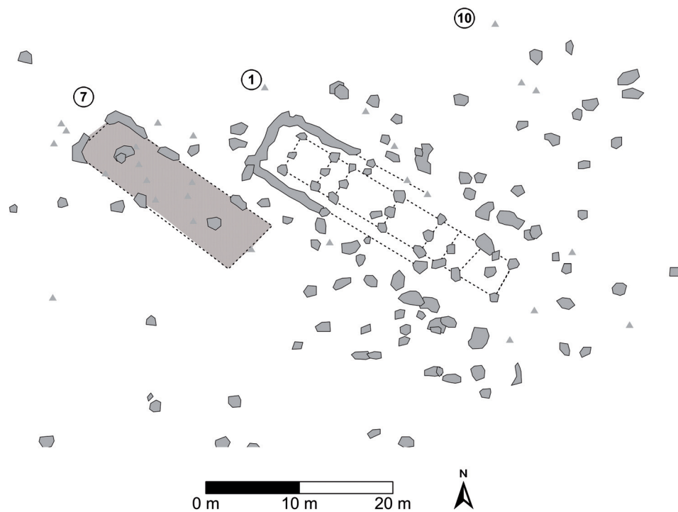
Abb. 2: Neolithische Siedlung, Frisange und Weiler-la-Tour, Luxembourg, archäologische Auswertung von Hausstandorten [Grafik: PZP GbR im Auftrag des Centre national de recherche archéologique, Bertrange, Luxembourg].
